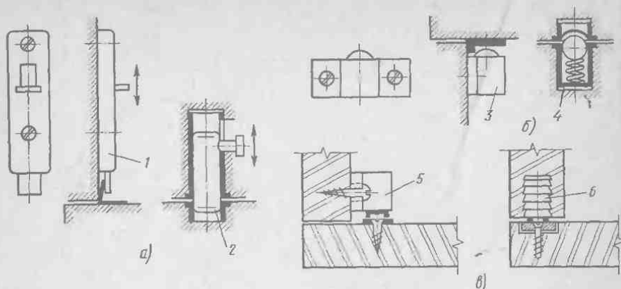
Рис. 76. Задвижки (а), защелки (б) и магнитные держатели (в):
