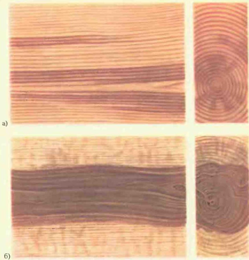
Рис. 21. Грибные ядровые пятна и полосы в древесине сосны (а) и березы (б)
