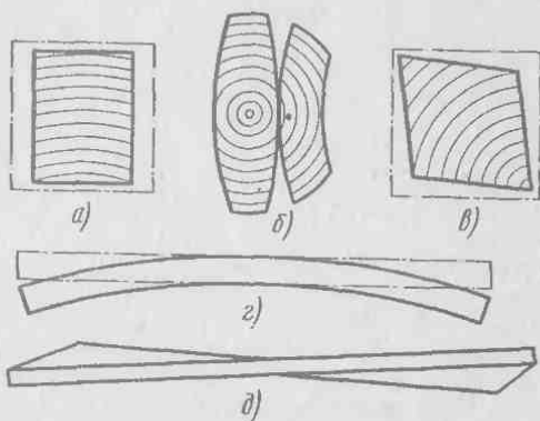
Рис. 11. Виды коробления:
