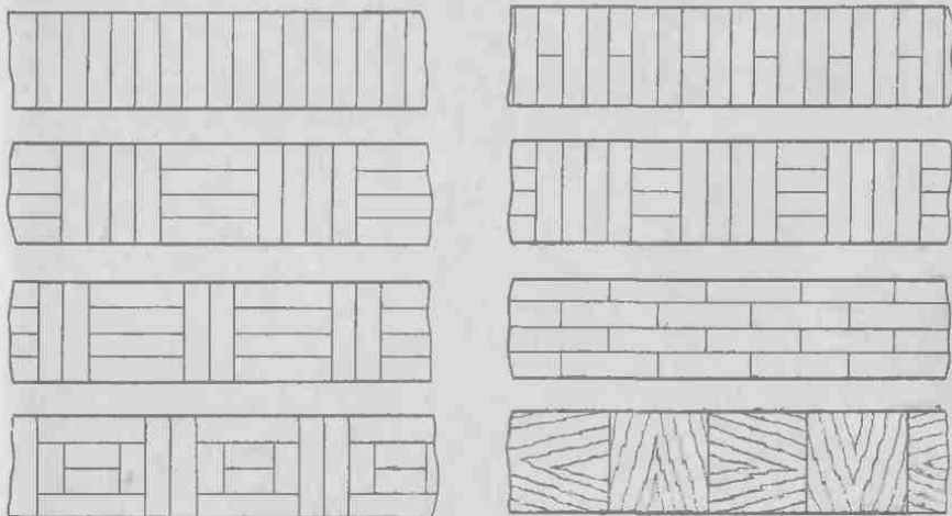
Рис. 52. Варианты рисунков планок и квадратов шпона паркетных досок
