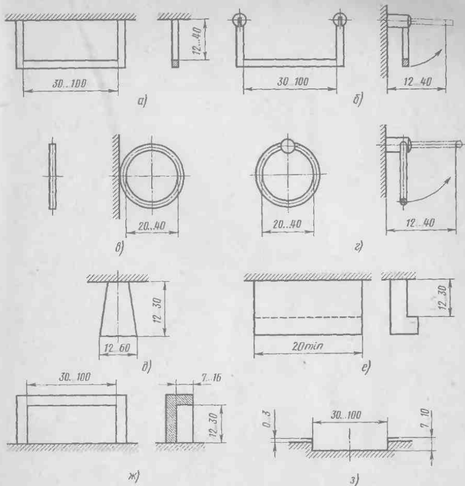
Рис. 78. Мебельные ручки:
