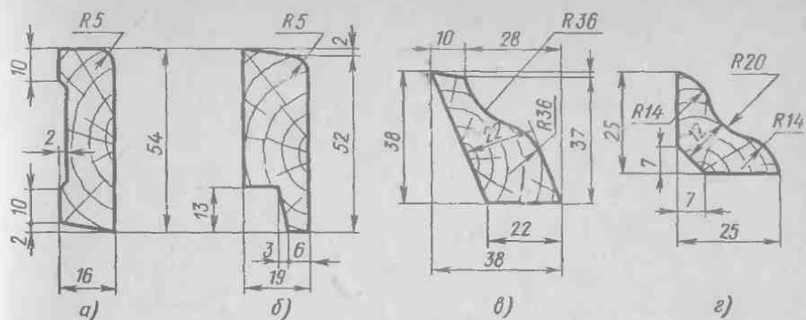
Рис. 58. Плинтусы типа 1 (а), типа 2 (б), типа 3 (в) и типа 4 (з)
