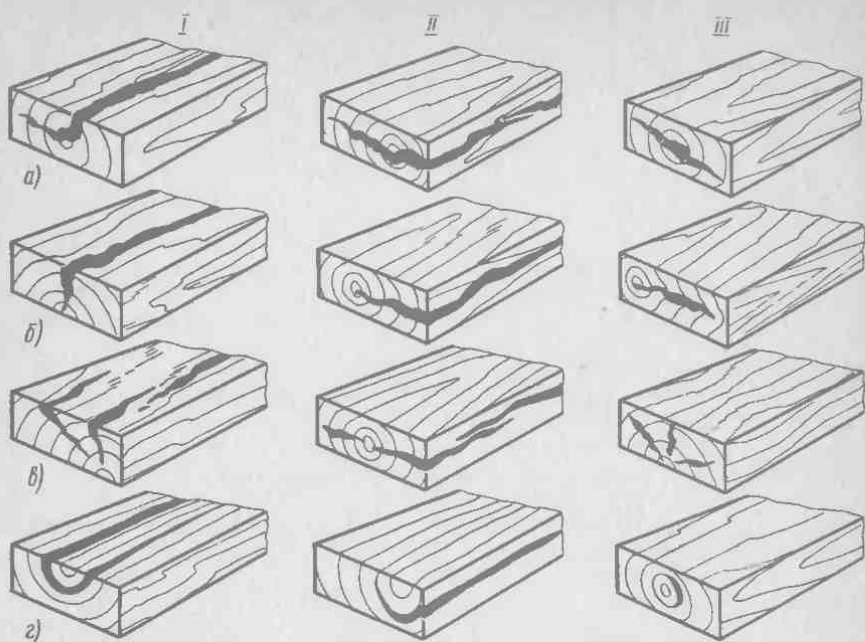
Рис. 17. Основные разновидности трещин в досках:
