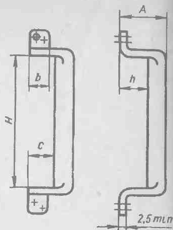
Рис. 68. Ручка-скоба
