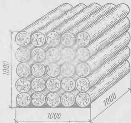
Рис. 32. Кубометр складочный
