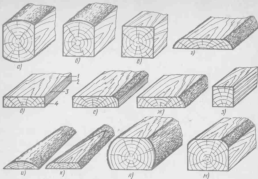
Рис. 33. Виды пилопродукции:
