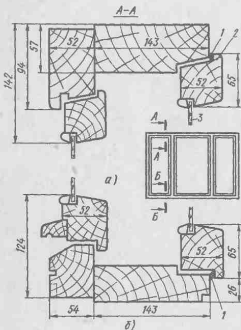
Рис. 44. Оконный блок с двойными раздельными переплетами с наплавом для общественных зданий:
