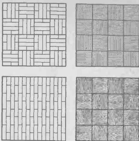
Рис. 54. Варианты рисунков планок и квадратов шпона паркетных щитов
