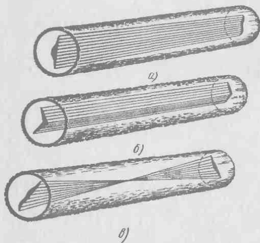
Рис. 18. Схемы метиковых трещин в круглых лесоматериалах:
