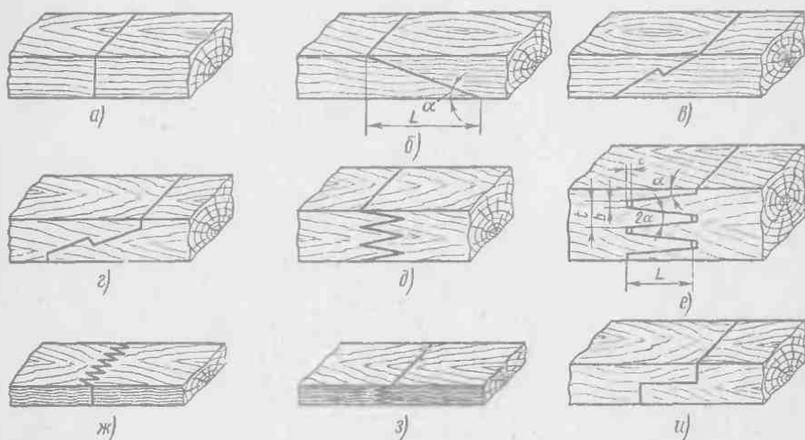
Рис. 36. Торцовые клеевые соединения заготовок: а — впритык, б — на ус, в — на ступенчатый ус, г — на ступенчатый ус с закруглением, д, е, ж, з — зубчатые клеевые соединения, и — ступенчатое клеевое соединение; \alpha — угол скоса, L — длина уса
