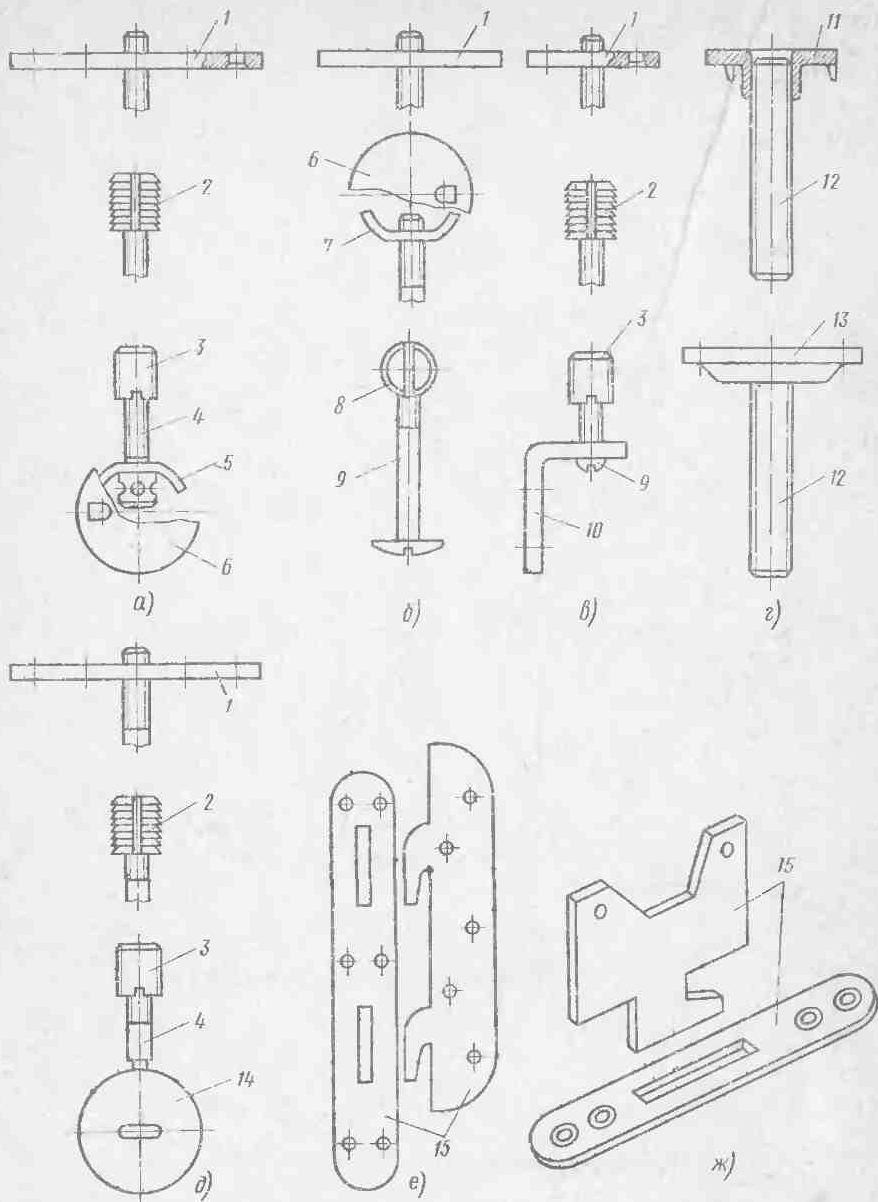
Рис. 74. Стяжки мебельные:
