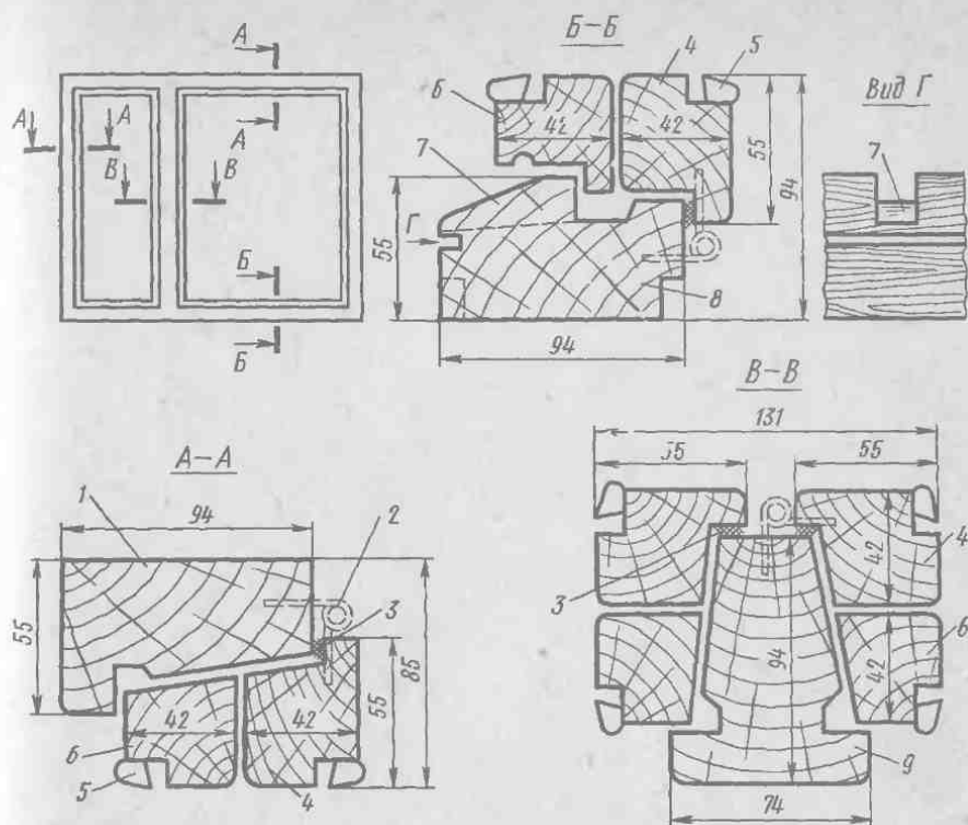
Рис. 45. Оконный блок со спаренными переплетами:
