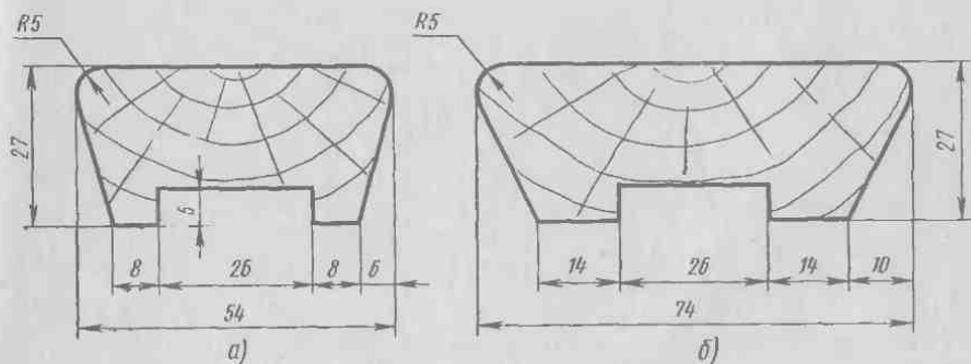
Рис. 60. Поручни типа 1 (а) и типа 2 (б)
