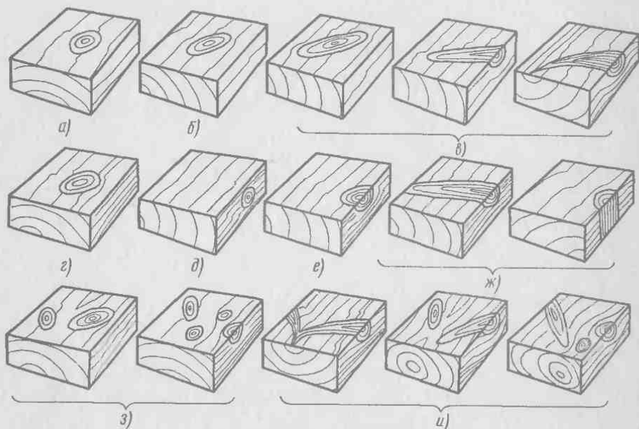
Рис. 12. Разновидности сучков:
