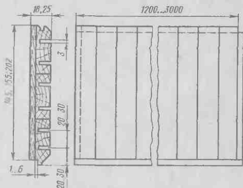
Рис. 51. Паркетная доска
