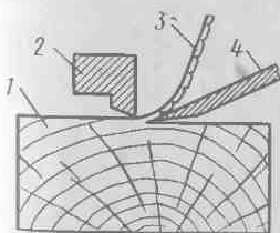
Рис. 39. Схема получения строганного шпона:
