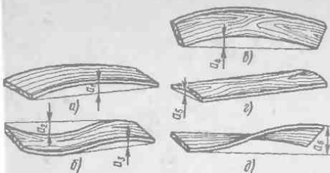
Рис. 27. Измерение покоробленности (схема):
