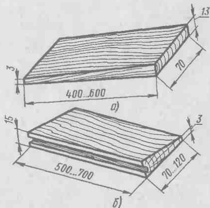
Рис. 63. Кровельные материалы:
