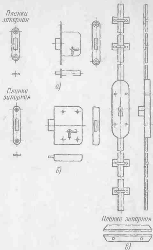
Рис 75. Мебельные замки:
