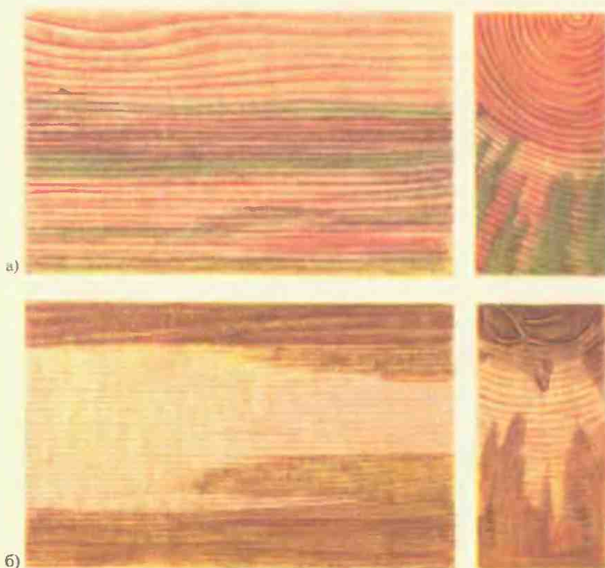
Рис. 24. Заболонные грибные окраски: а — синева (розовая и коричневая окраски), б — побурение
